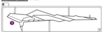
Rパーツ×1 (PS製)
