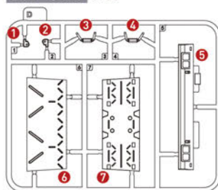
Dパーツ×1 (PS製)
