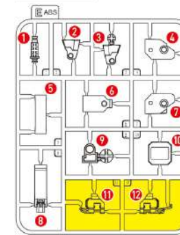
Eパーツ×1 (ABS製)
