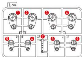
Lパーツ×1 (ABS製)
